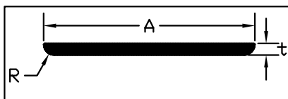
נספח פינה אחד מעוגלת FLAT PROFILE WITH ROUND ONE CORNER
